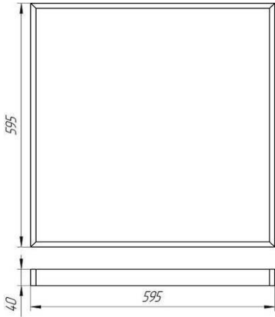
Рисунок 1. Габаритный чертеж Econex Office 595x595 G2 EM
