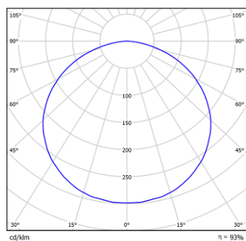
Рисунок 2. КСС типа Д (косинусная)
