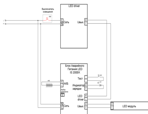
Рисунок 3. Схема подключение светильника Econex Office EGr 1188x288 EM
