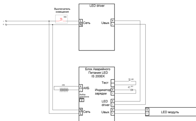
Рисунок 3. Схема электрическая
