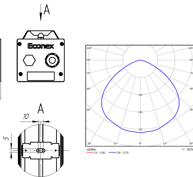
Рисунок 2. КСС типа Д120
