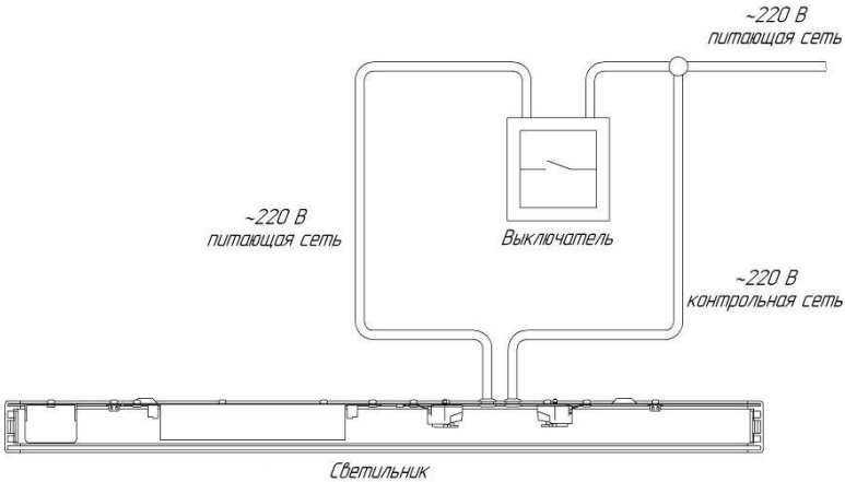
Рисунок 3. Схема подключение светильника 1195x295 G2 EM
