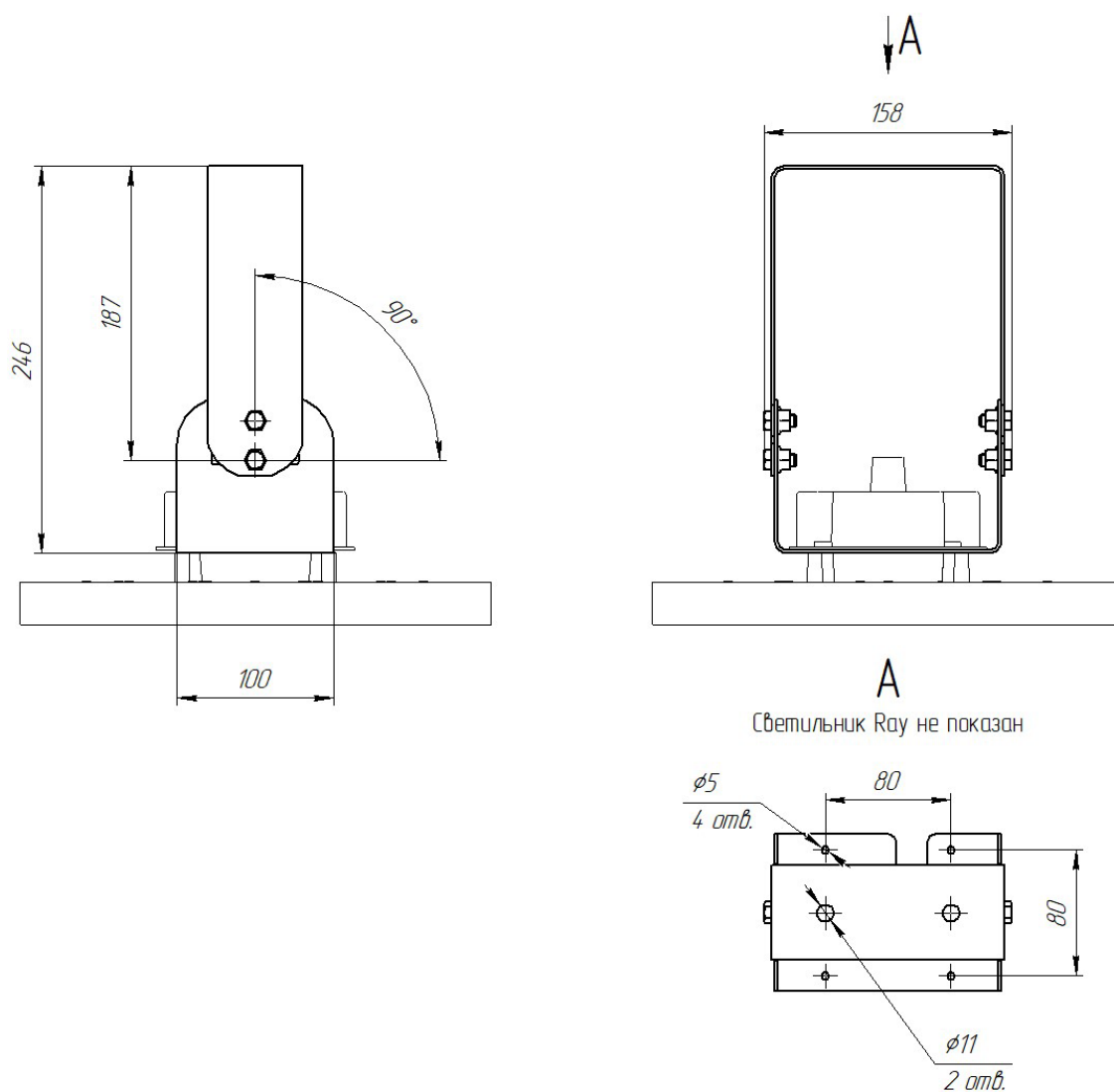
Рис.1 Установка комплекта.
