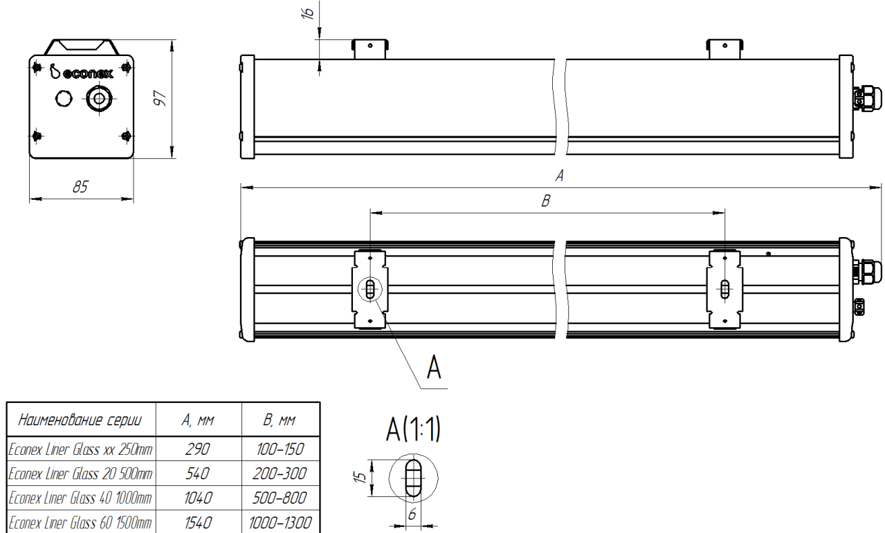
Рисунок 1. Габаритный чертеж Econex Liner
