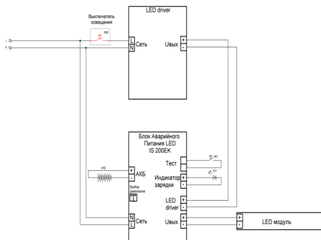
Рисунок 2. Схема подключения светильника Econex Office E 1195x295 EM
