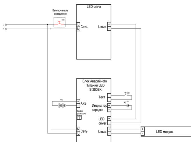
Рисунок 2. Схема подключения светильника Esonex Office E 1195x595 EM
