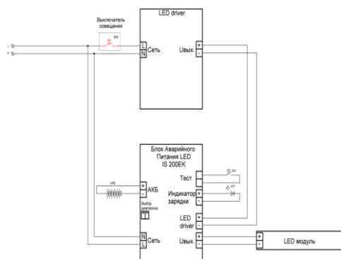
Рисунок 4. Схема подключения светильника Econex Office E 595x595 EM
