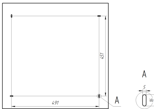
Рисунок 2. Расположение установочных отверстий на корпусе светильника Econex Office E 595x595 для накладного монтажа.
