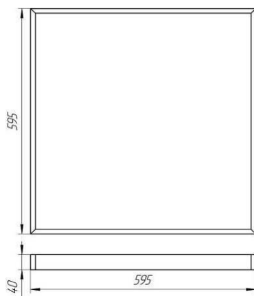
Рисунок 1. Габаритный чертеж Econex Office E 595x595
