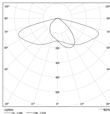
Рисунок 5. КСС типа Ш2 (Широкая боковая)
