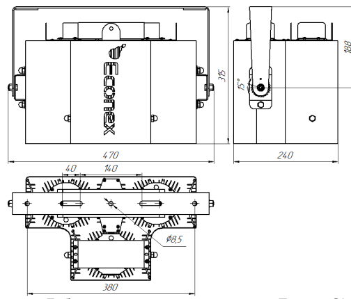
Рисунок 4. Габаритный чертеж светильника Econex SkyX 360
