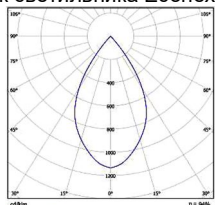
Рисунок 8. КСС типа G60 (глубокая)
