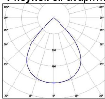
Рисунок 7. КСС типа Д (косинусная)
