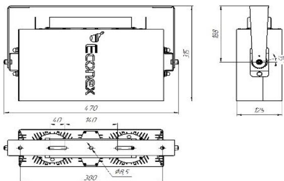
Рисунок 5. Габаритный чертеж светильника Ecomex SkyX 240
