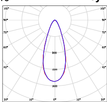
Рисунок 9. КСС типа K25 (концентрированная)
