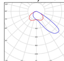
Рисунок 11. КСС типа А (асимметричная)
