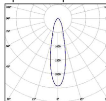
Рисунок 10. КСС типа K23 (концентрированная)
