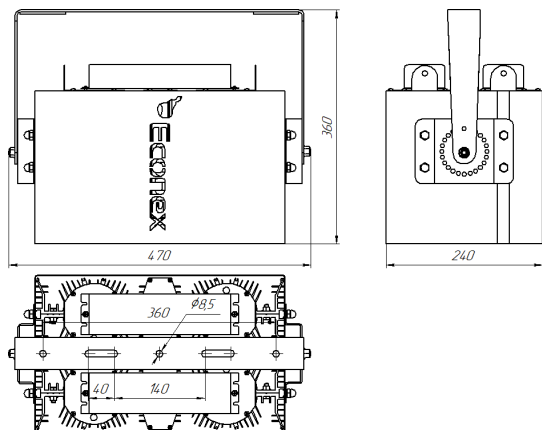
Рисунок 3. Габаритный чертеж светильника Econex SkyX 480
