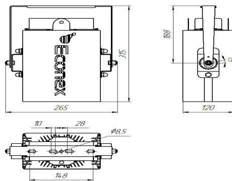
Рисунок 6. Габаритный чертеж светильника Ecomex SkyX 120
