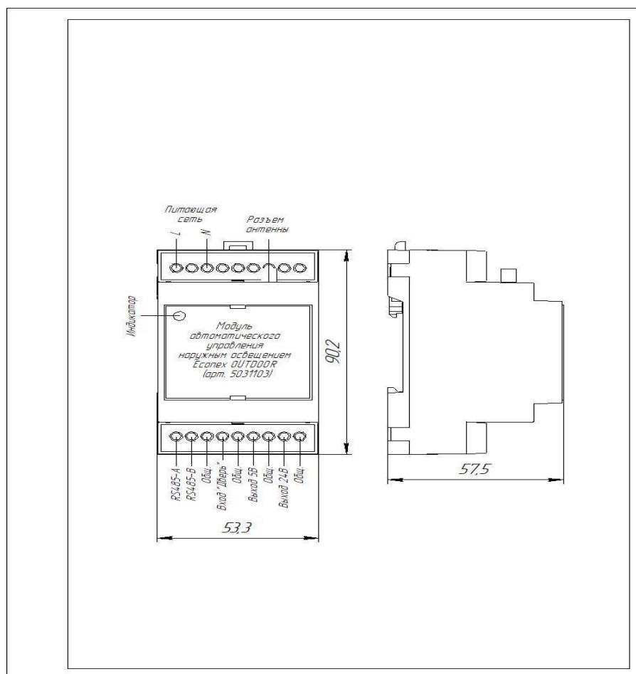
Рисунок 1. Габаритный чертеж и расположение контактов
