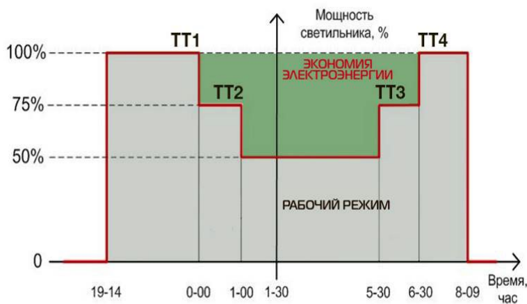
Рисунок 9. Графика работы светильника с функцией Ночной диммер
