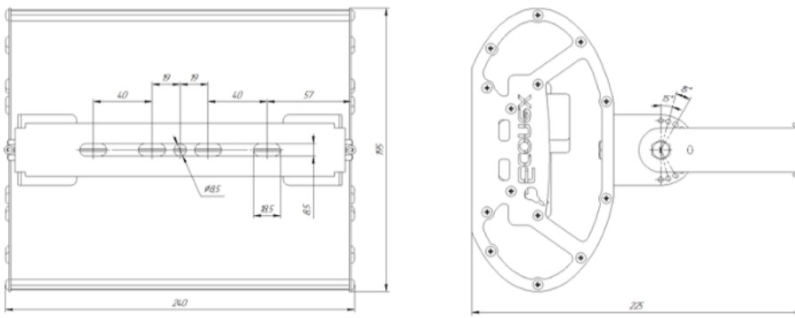
Рисунок 1. Габаритный и присоединительный чертеж светильника Ecomex Board 24
