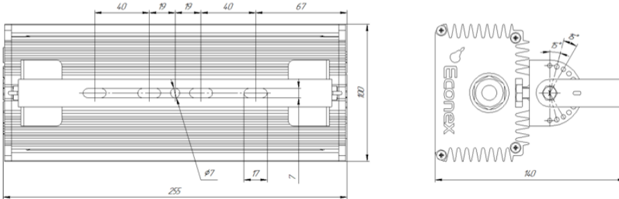
Рисунок 1. Габаритный и присоединительный чертеж светильника Ecomex Board 24
